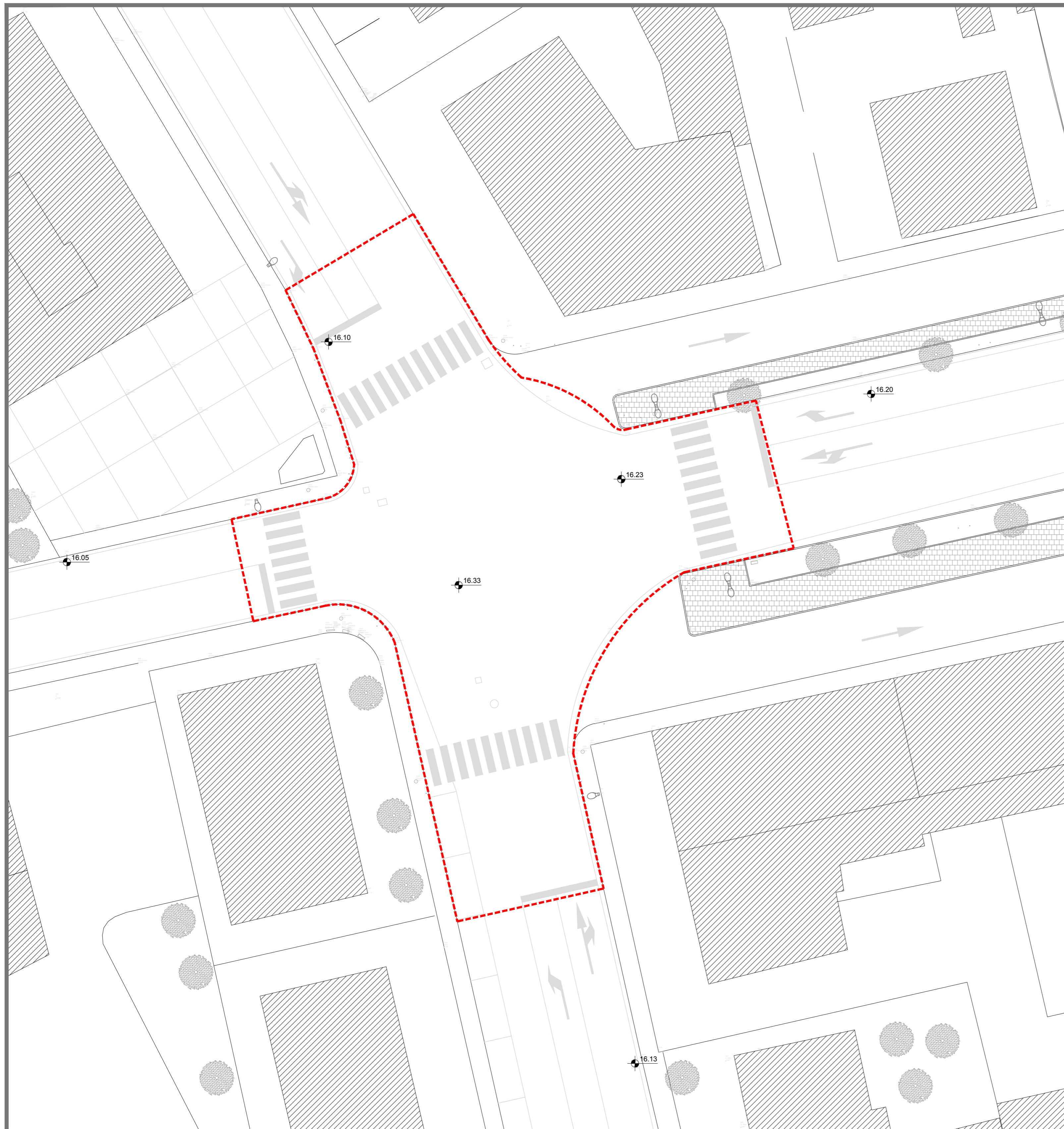
RILIEVO AREA INTERVENTO - scala 1:200
