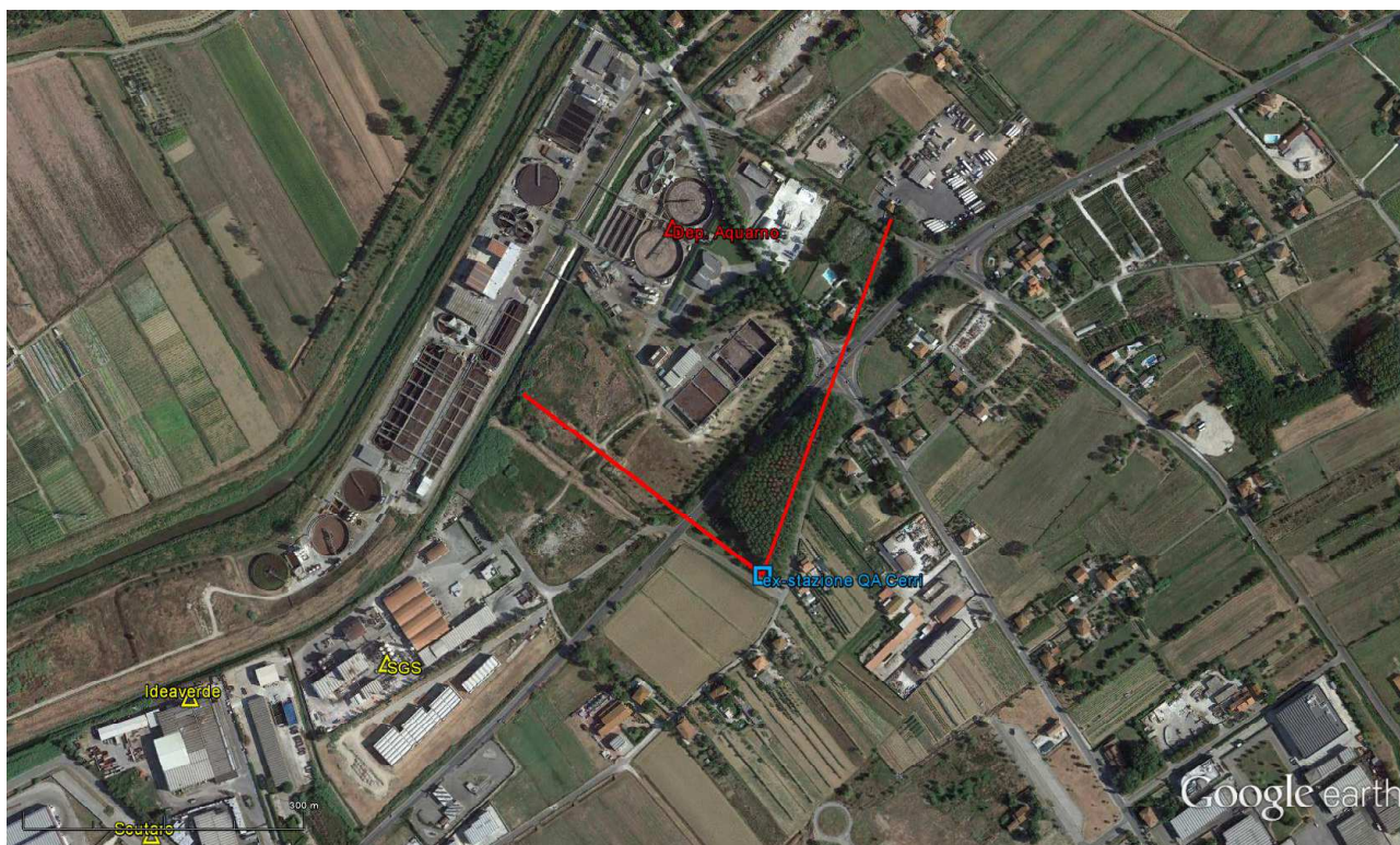
Figura 15 - Settore di provenienza del vento (307-20 °N) che pone il laboratorio mobile sottovento alle vasche OMO1 e OMO2 del depuratore Aquarno (immagine Google Earth ©).
