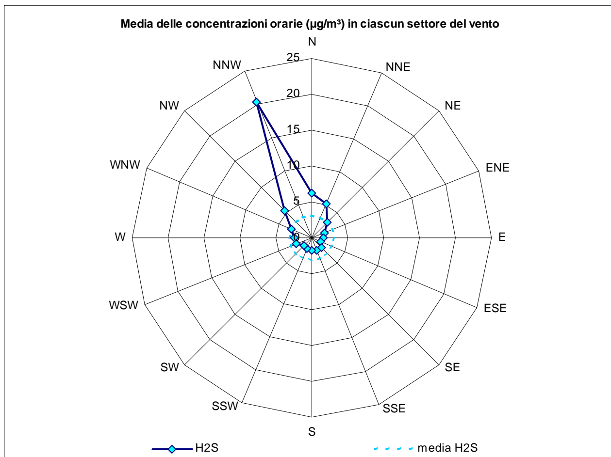
Figura 6 - Media delle concentrazioni ( \mu\text{g}/\text{m}^3 ) di \text{H}_2\text{S} in ciascuno dei 16 settori di provenienza del vento. E' indicata anche la media complessiva nel periodo 24.7.2013-10.2.2014 ( 3.1 \mu\text{g}/\text{m}^3 ).
