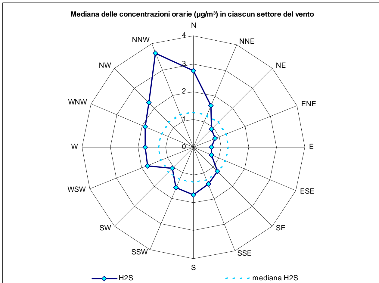
Figura 5 - Mediana delle concentrazioni ( \mu\text{g}/\text{m}^3 ) di \text{H}_2\text{S} in ciascuno dei 16 settori di provenienza del vento. E' indicata anche la mediana complessiva nel periodo 24.7.2013-10.2.2014 ( 1.3 \mu\text{g}/\text{m}^3 ).
