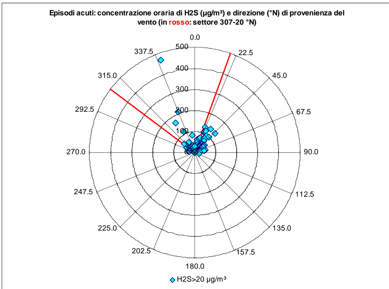
Figura 16 – Diagramma polare delle concentrazioni orarie di H 2 S (µg/m 3 ) negli 84 episodi acuti, in relazione alla direzione di provenienza del vento (°N). Le righe rosse delimitano il settore di direzione del vento (307-20 °N) per il quale il laboratorio mobile è stato considerato sottovento alle vasche OMO1 e OMO2 del depuratore Aquarno.
