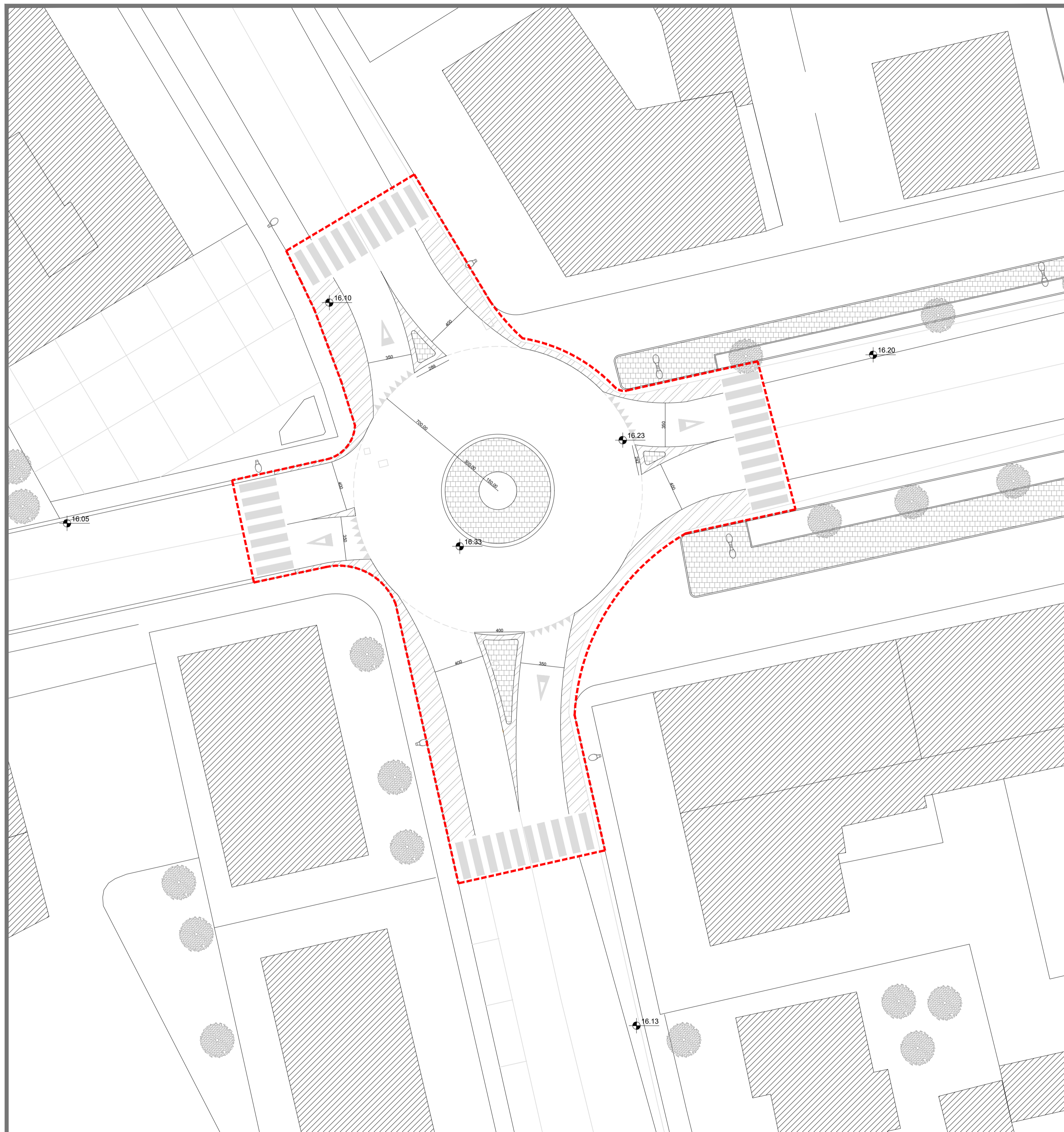
PLANIMETRIA DI PROGETTO - scala 1:200
