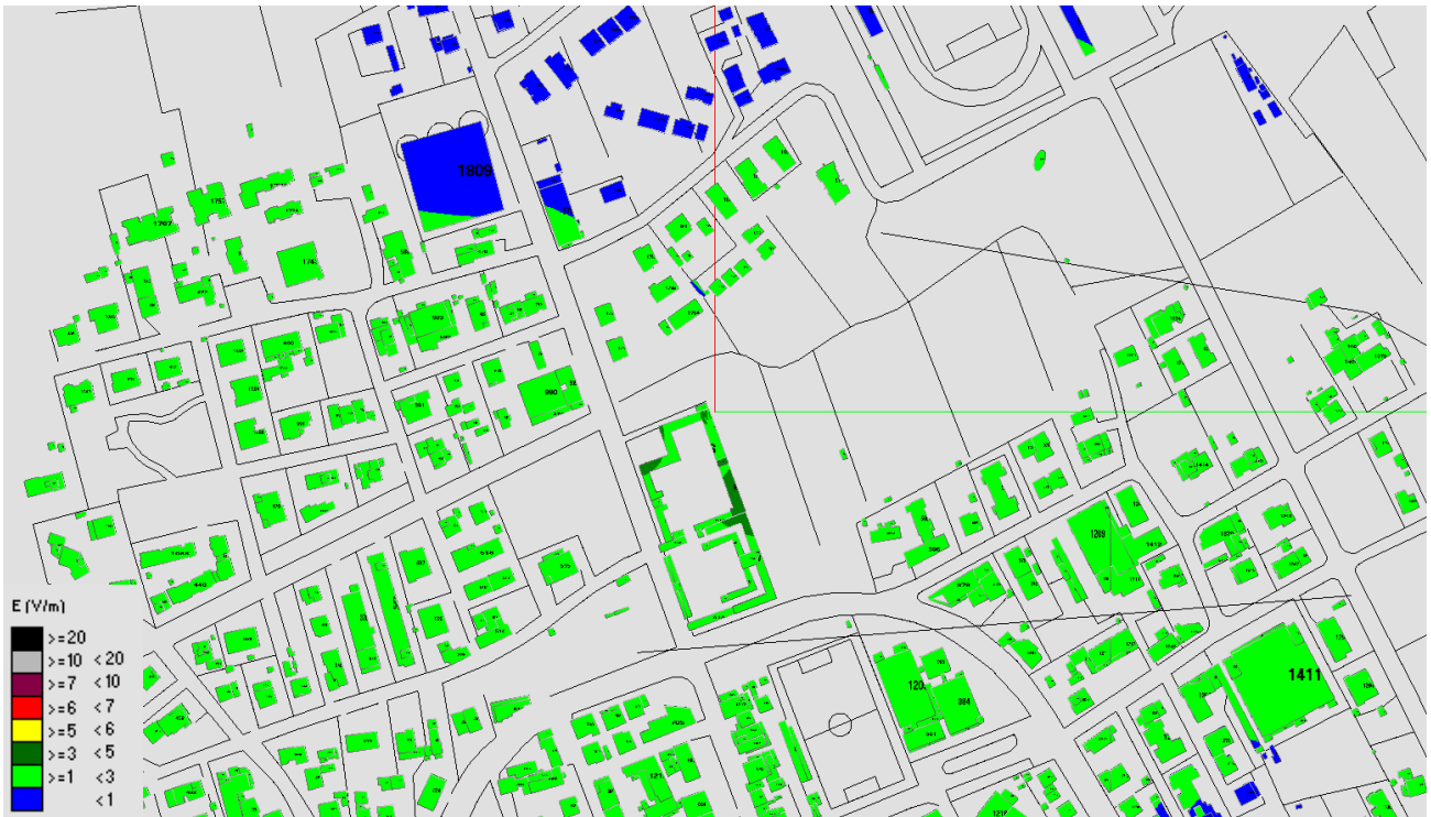
Fig. 27 Impatto elettromagnetico – zona Cimitero Comunale – Vista dall'alto
