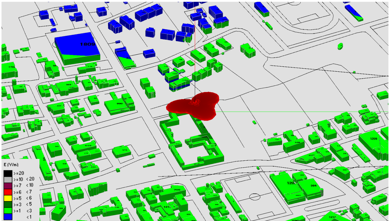
Fig. 26 Impatto elettromagnetico – zona Cimitero Comunale – 0°/Nord
