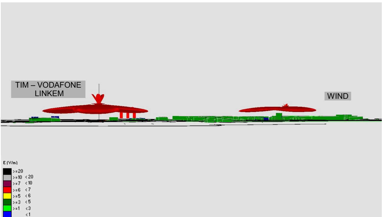
Fig. 25 Impatto elettromagnetico – zona Via dei Tavi e Centrale Enel – Ipotesi 2 – Vista Laterale
