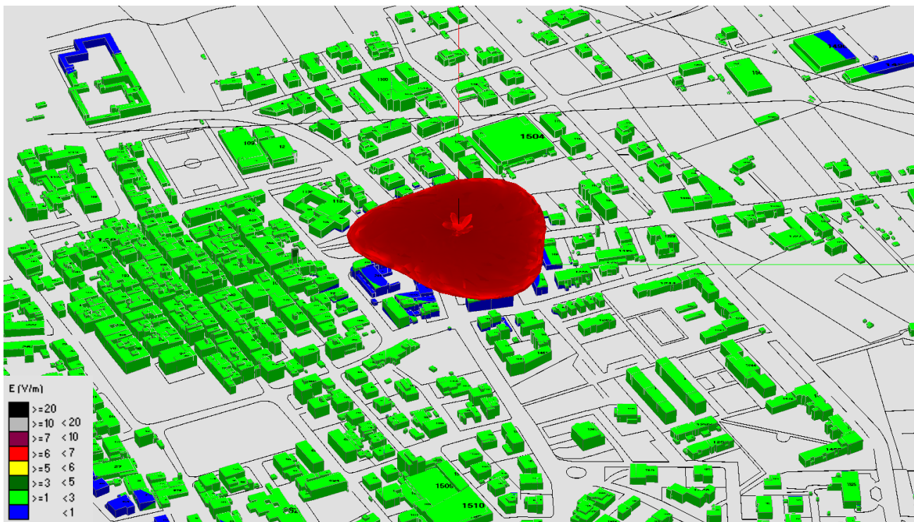
Fig. 13 Impatto elettromagnetico – zona Castelfranco di Sotto Centro – 0°/Nord
