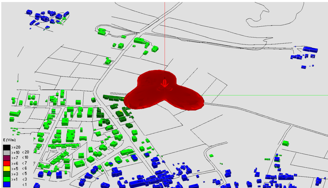
Fig. 1 Impatto elettromagnetico – zona Località Orentano Via Ponticelli – 0°/Nord
