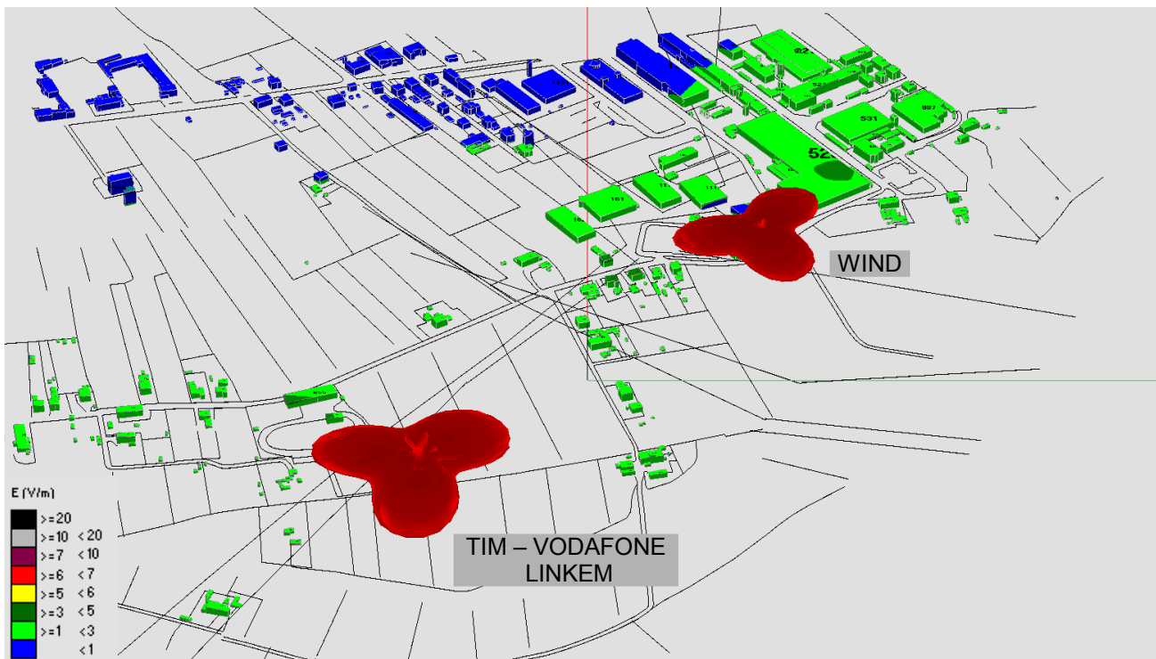
Fig. 21 Impatto elettromagnetico – zona Via dei Tavi e Centrale Enel – Ipotesi 2 – 0°/Nord
