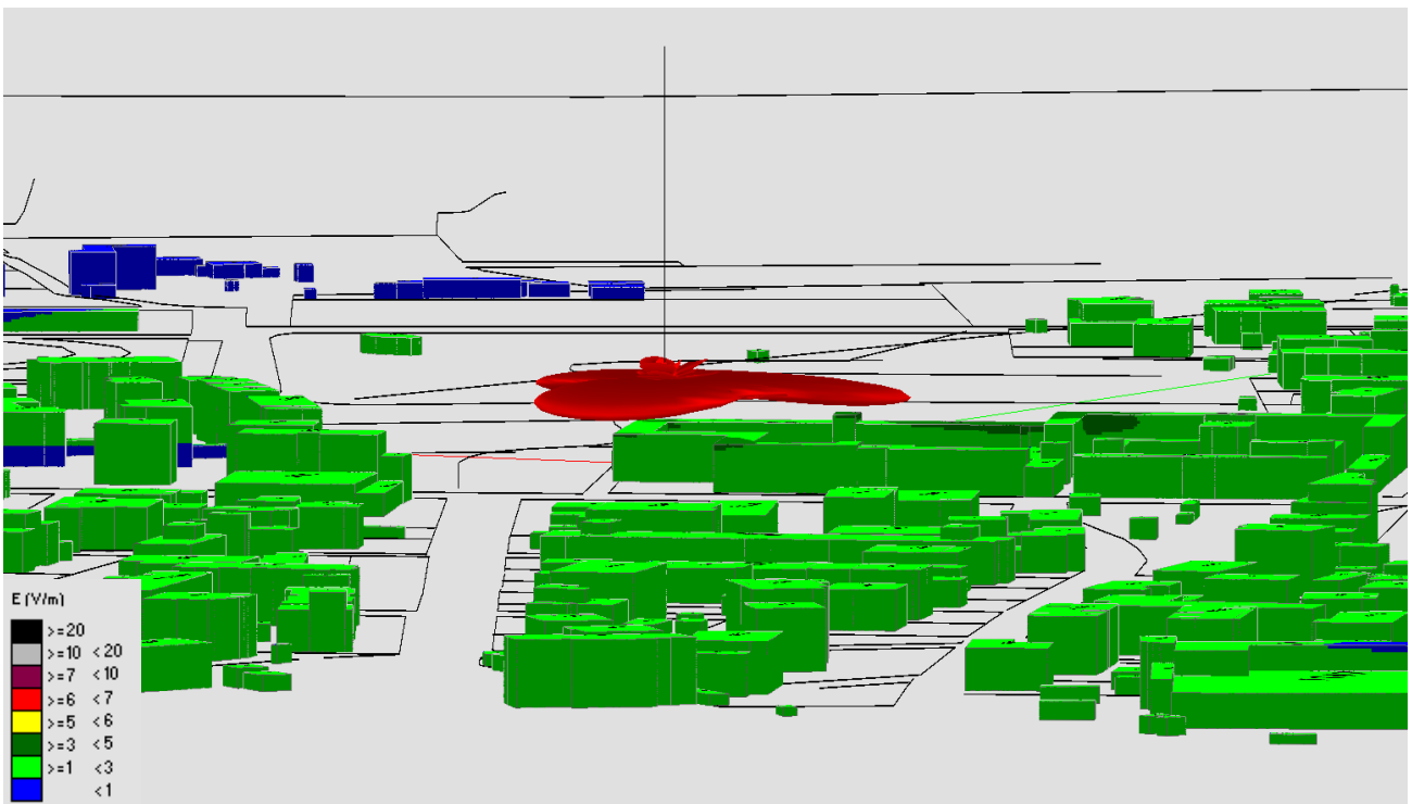
Fig. 28 Impatto elettromagnetico – zona Cimitero Comunale – Vista Laterale
