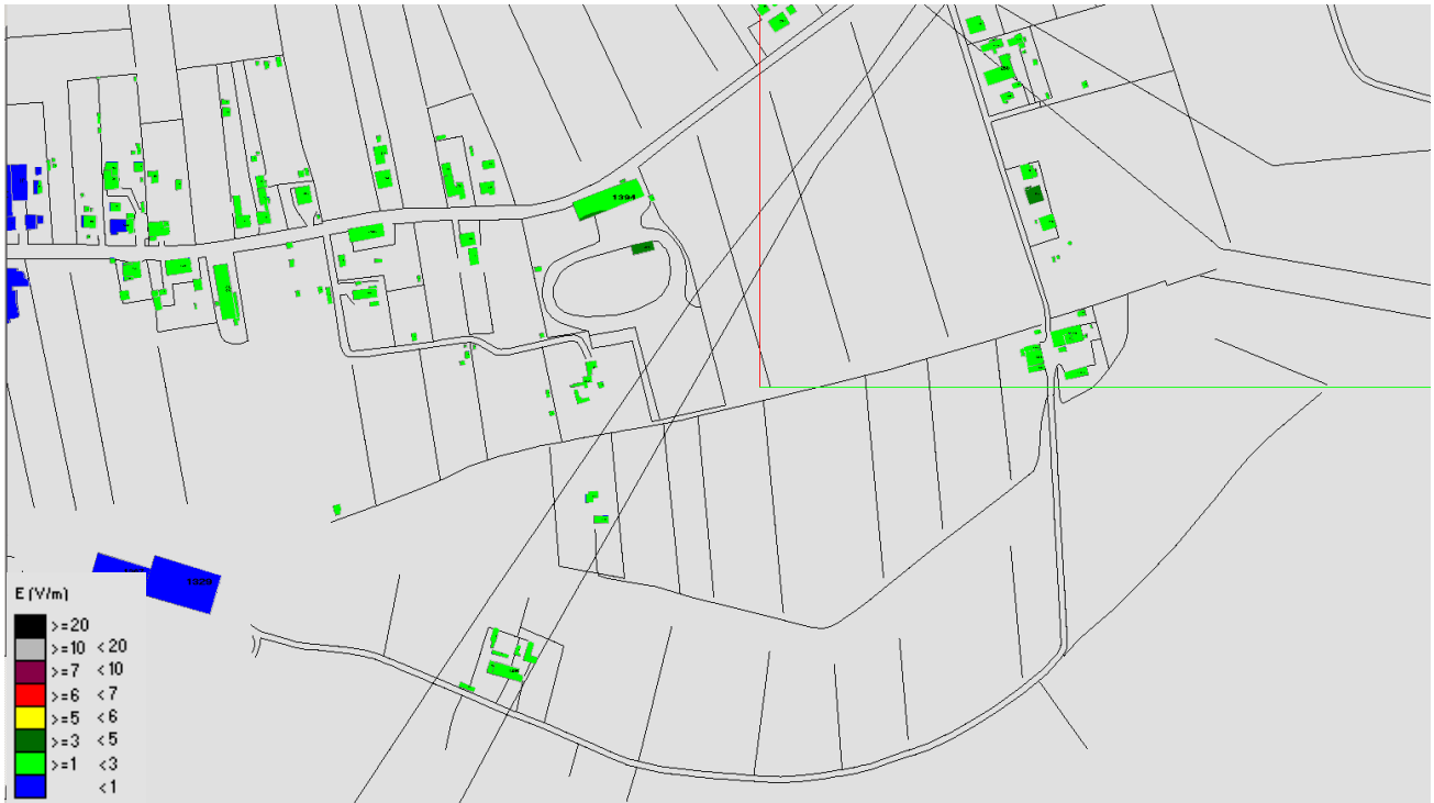
Fig. 19 Impatto elettromagnetico – zona Via dei Tavi e Centrale Enel – Ipotesi 1 – Vista dall'alto
