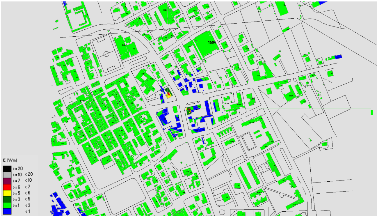
Fig. 14 Impatto elettromagnetico – zona Castelfranco di Sotto Centro – Vista dall'alto
