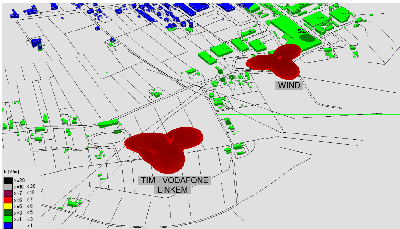
Fig. 16 Impatto elettromagnetico – zona Via dei Tavi e Centrale Enel – Ipotesi 1 – 0°/Nord
