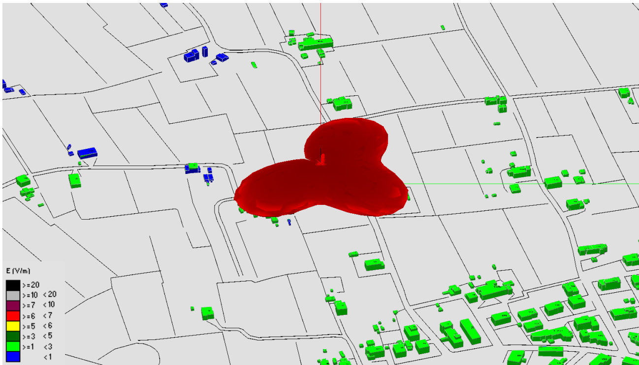
Fig. 7 Impatto elettromagnetico – zona Via dell'Iserone – 0°/Nord
