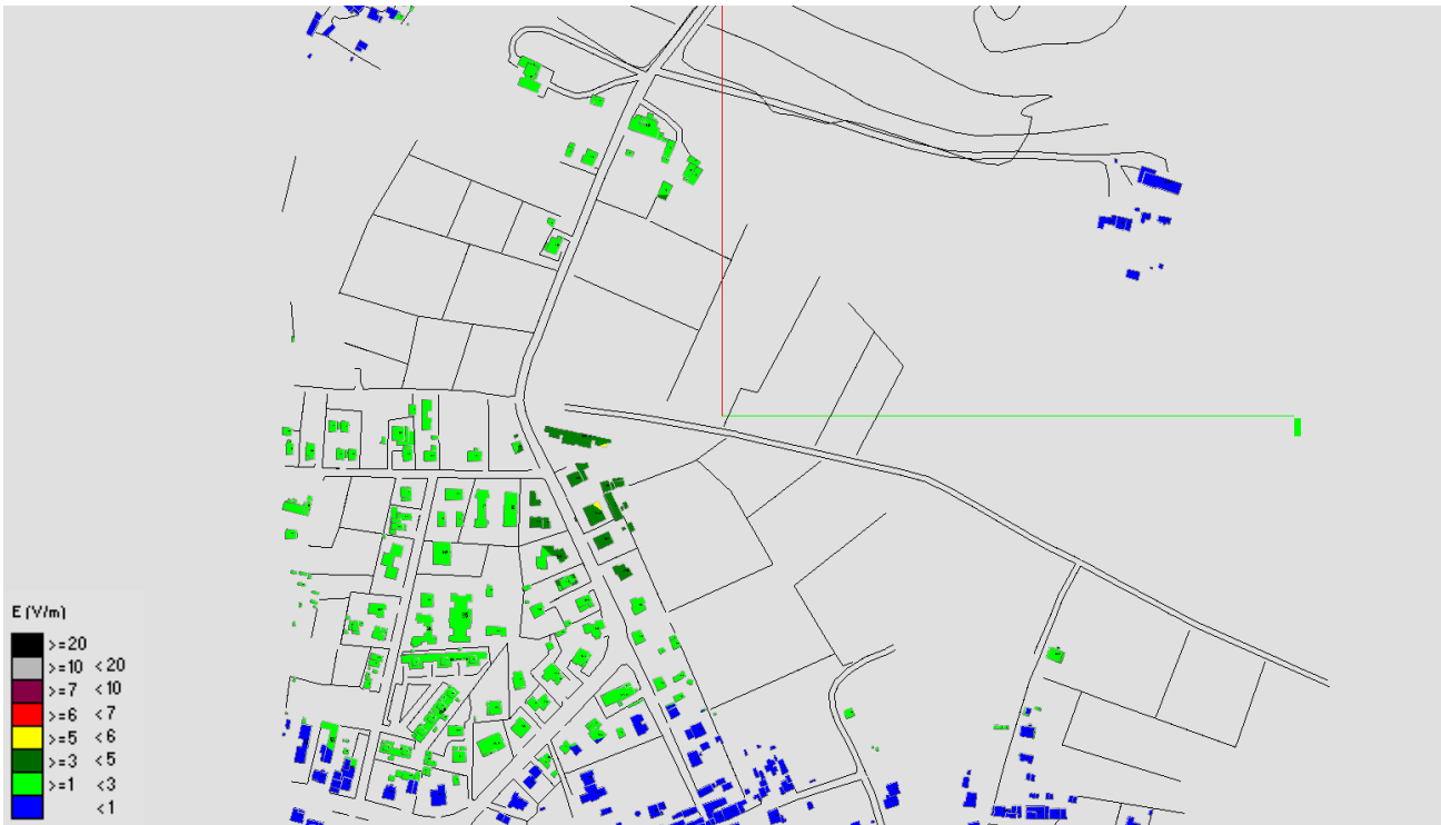
Fig. 2 Impatto elettromagnetico – zona Località Orentano Via Ponticelli – Vista dall'alto
