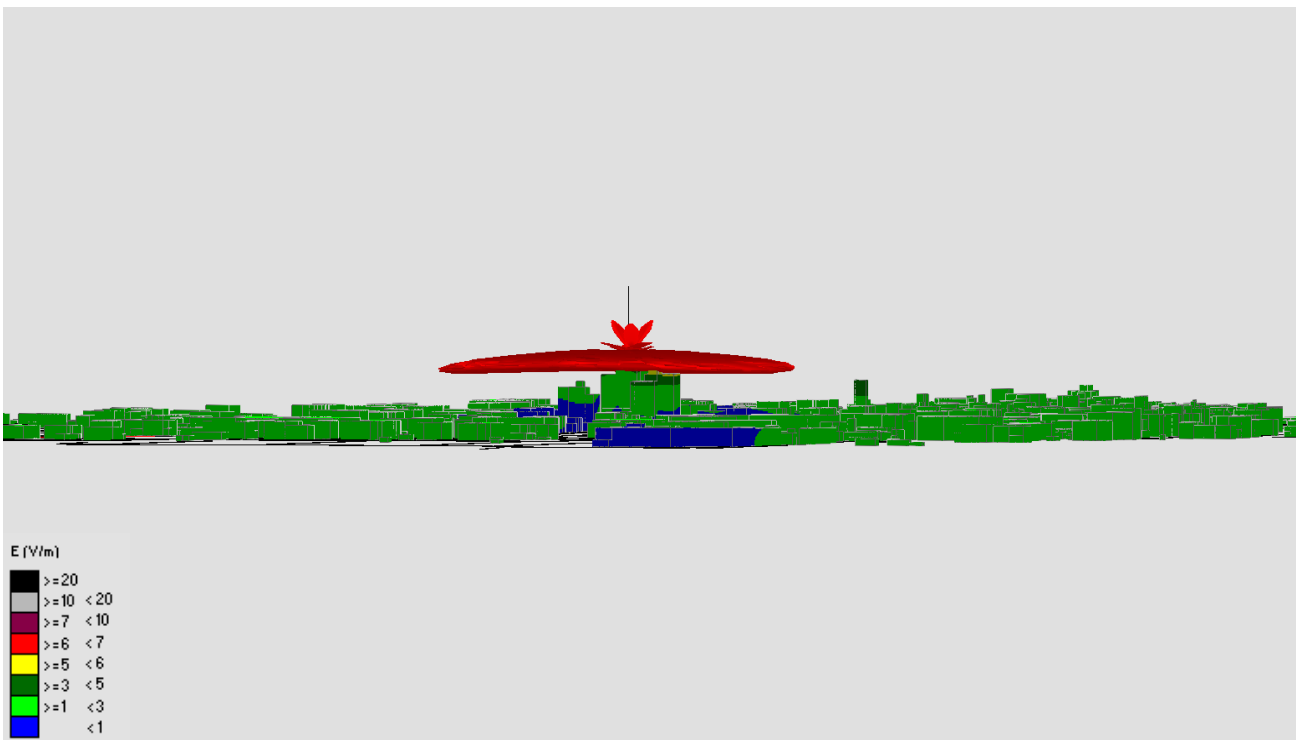
Fig. 15 Impatto elettromagnetico - zona Castelfranco di Sotto Centro - Vista Laterale
