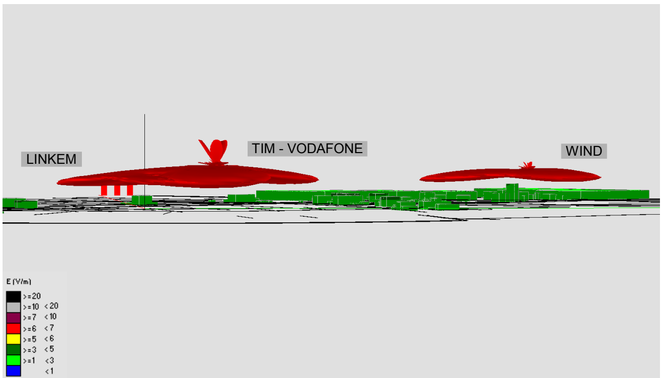
Fig. 20 Impatto elettromagnetico – zona Via dei Tavi e Centrale Enel – Ipotesi 1 – Vista Laterale
