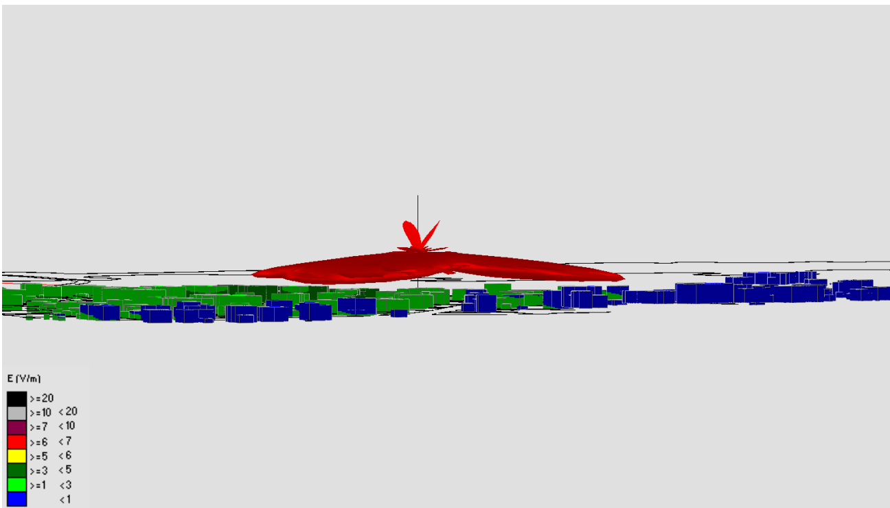
Fig. 3 Impatto elettromagnetico – zona Località Orentano Via Ponticelli – Vista Laterale
