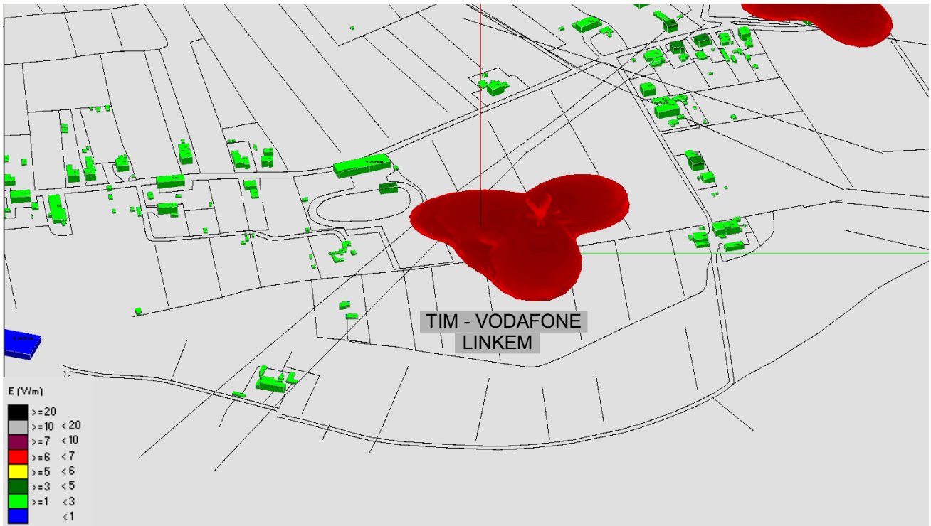
Fig. 17 Impatto elettromagnetico – zona Via dei Tavi e Centrale Enel – Ipotesi 1 – 0°/Nord
