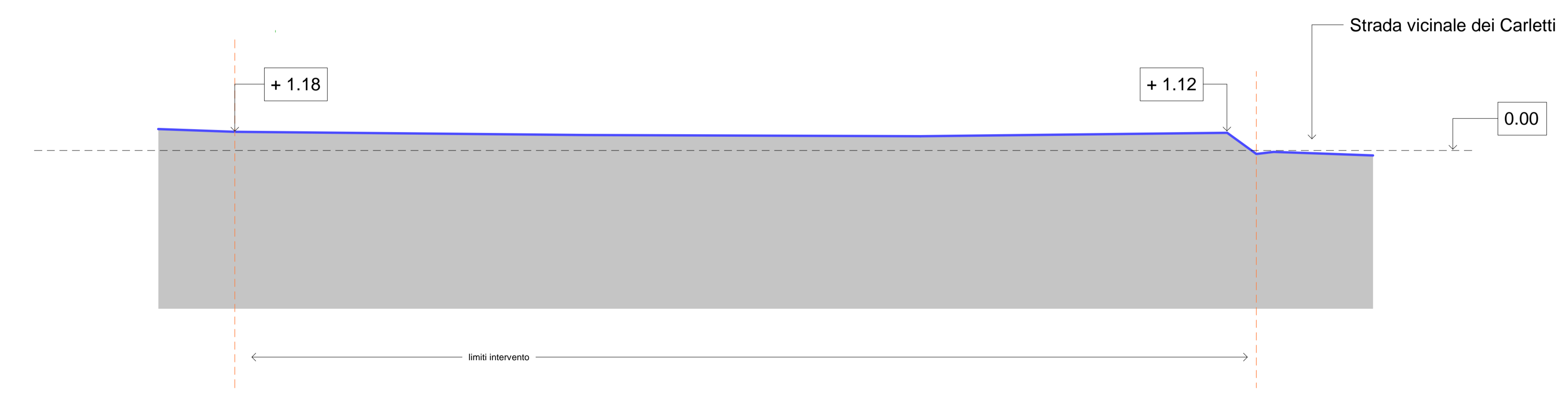
Sez. D-D'
