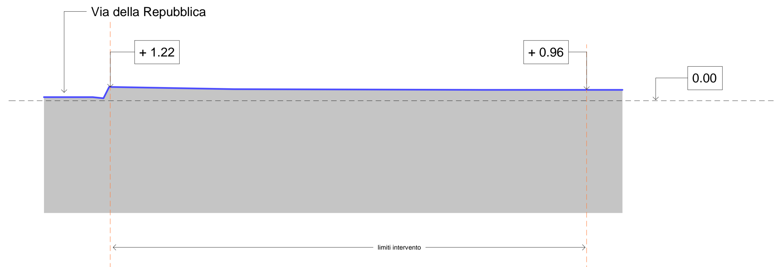
Sez. A-A'
