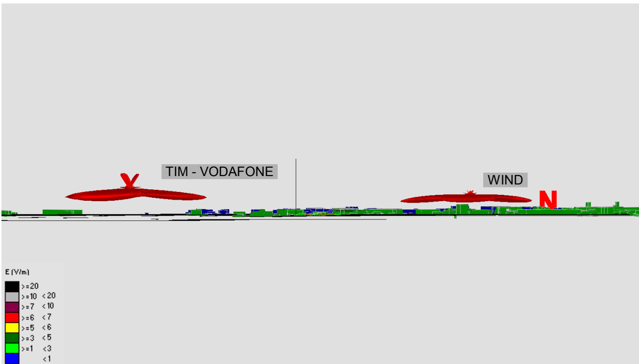
Fig. 19 Impatto elettromagnetico – zona Via dei Tavi e Centrale Enel – Vista Laterale
