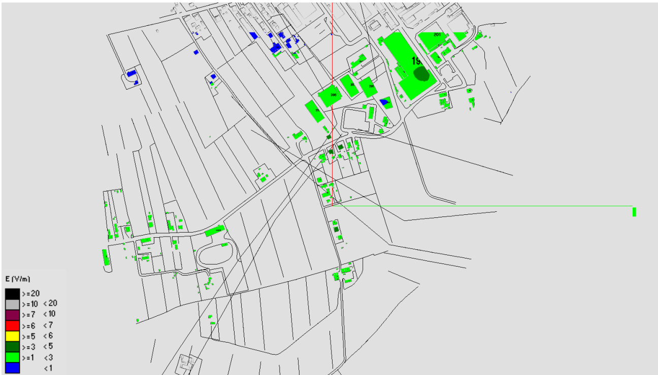
Fig. 18 Impatto elettromagnetico – zona Via dei Tavi e Centrale Enel – Vista dall'alto
